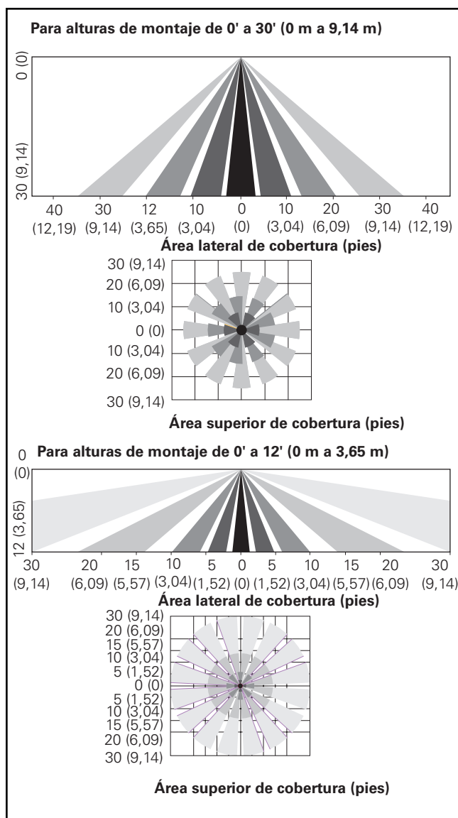
Figura 1. Patrones de detección del sensor de ocupación
