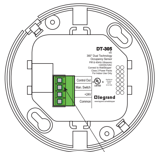
Wiring terminals
